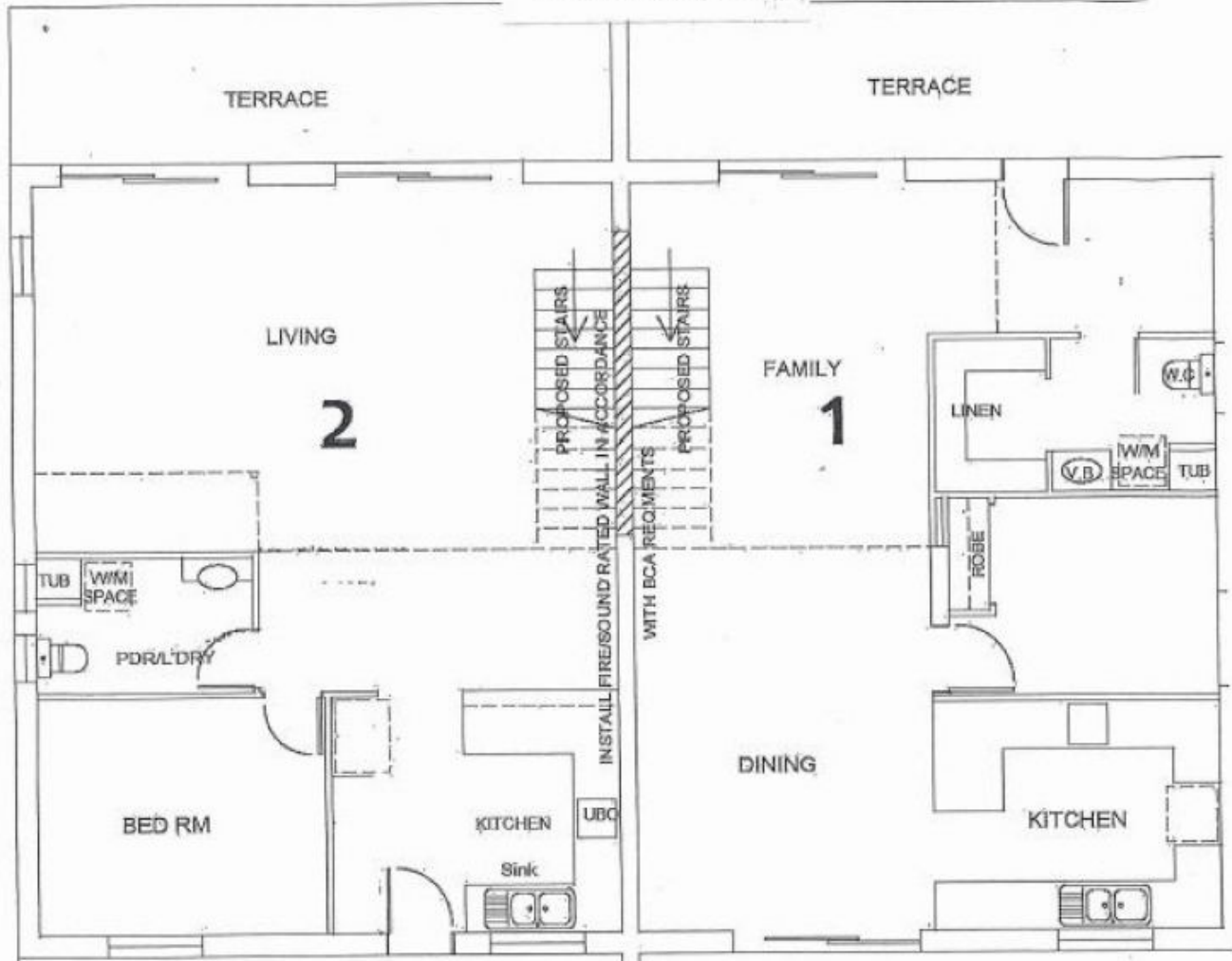
65-Bentlnck-St-Lower-Level.jpg
